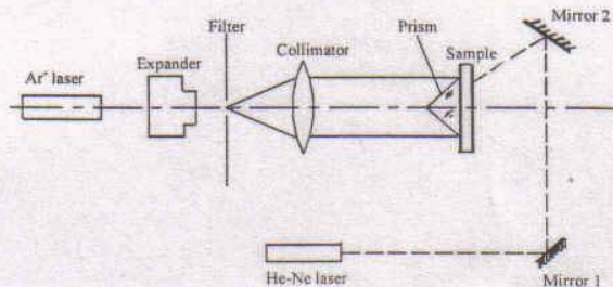
图 2 全息记录装置
