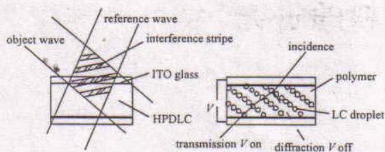
图 1 HPDLC 形成及工作原理
